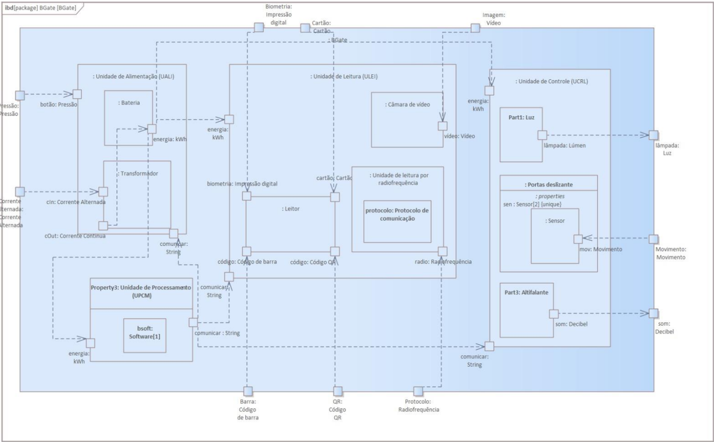
S2: Diagrama interno de blocos representando uma BGate e alinhado com o respetivo diagrama de blocos
